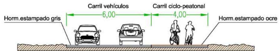
Sección transversal conexión paseo litoral con pasarela Rambla Cervera
