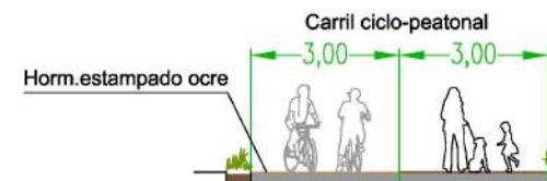
Sección transversal paseo litoral
