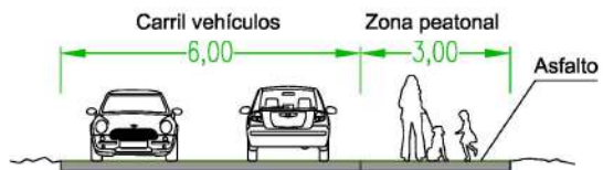
Sección transversal Avgda. de les Illes Balears
